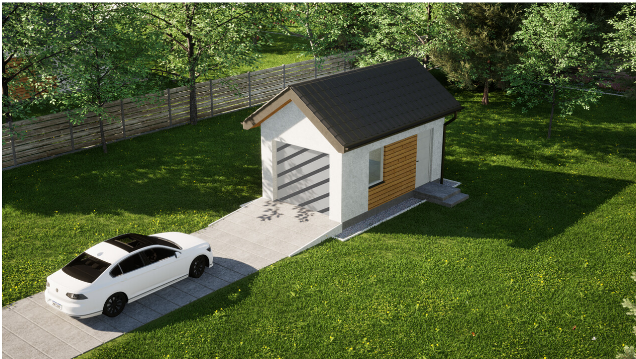
Garaz ERDOL G1 - Wersja prawa - Układ kalenicy prostopadły z dachem dwuspadowym o kącie nachylenia 35 stopni - Bez bramy - Białe
